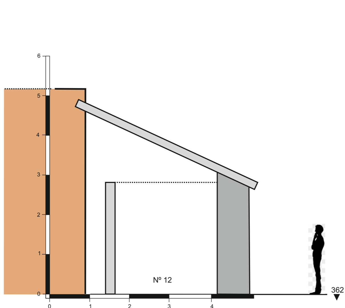
PERFIL 1: EDIFICIO ADOSADO EXTRAMUROS. LIENZO EXTERNO DE LA MURALLA Y SECCIÓN DEL SOLAR N° 12 DE LA CALLE DE LA MURALLA (SONDEO ARQUEOLÓGICO 1).
