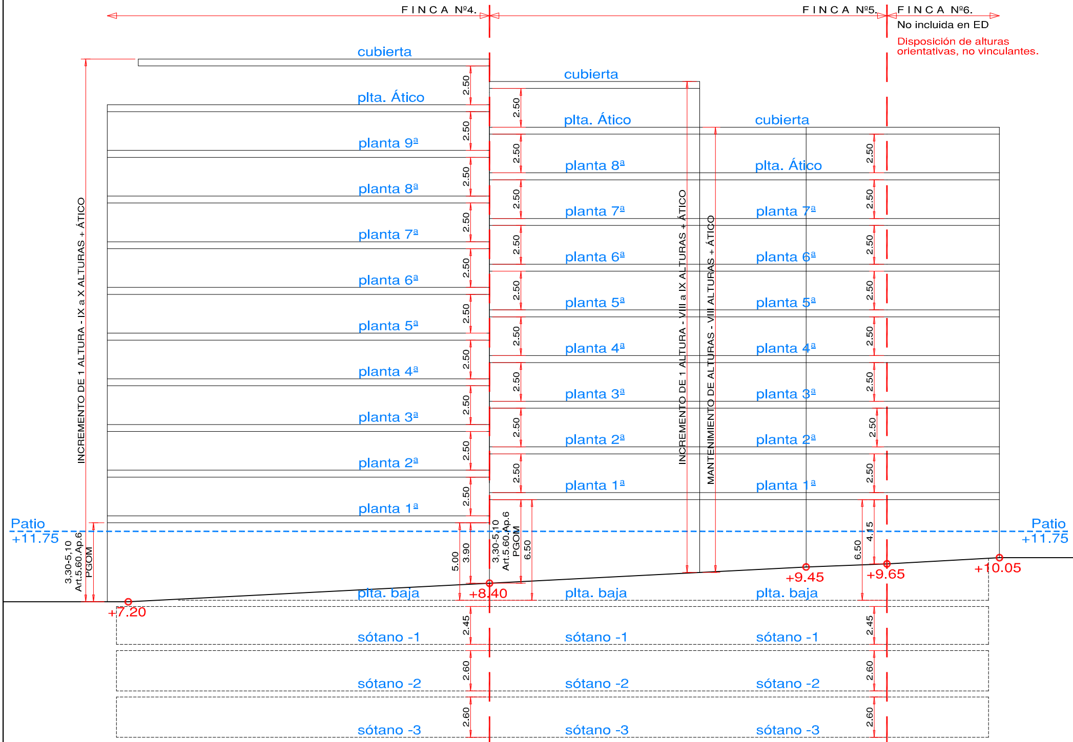
ESQUEMA DE ALZADO a C/ JOSÉ CUETO.
