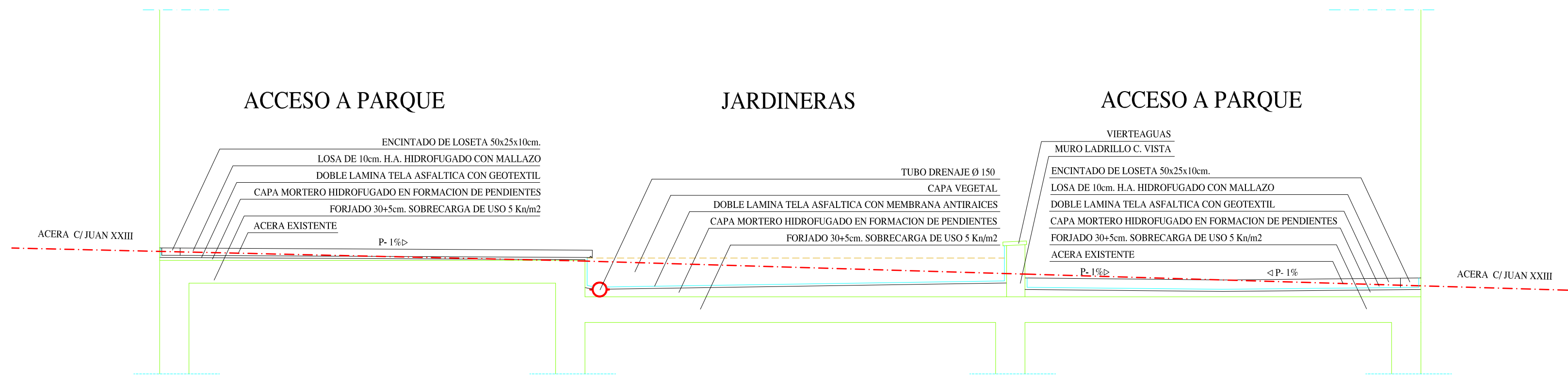
DETALLE SECCION TRANSVERSAL T-1 escala 1/50
