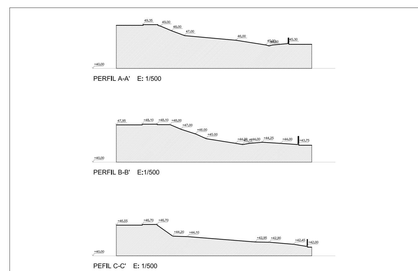
PERFILES TRANSVERSALES E:1/500
