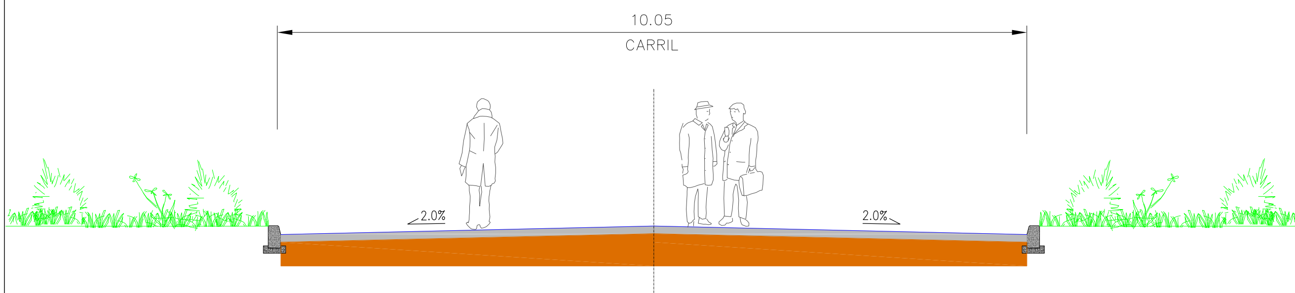
SECCION TIPO VIAL PEATONAL Y VIAL COMPARTIDO A
