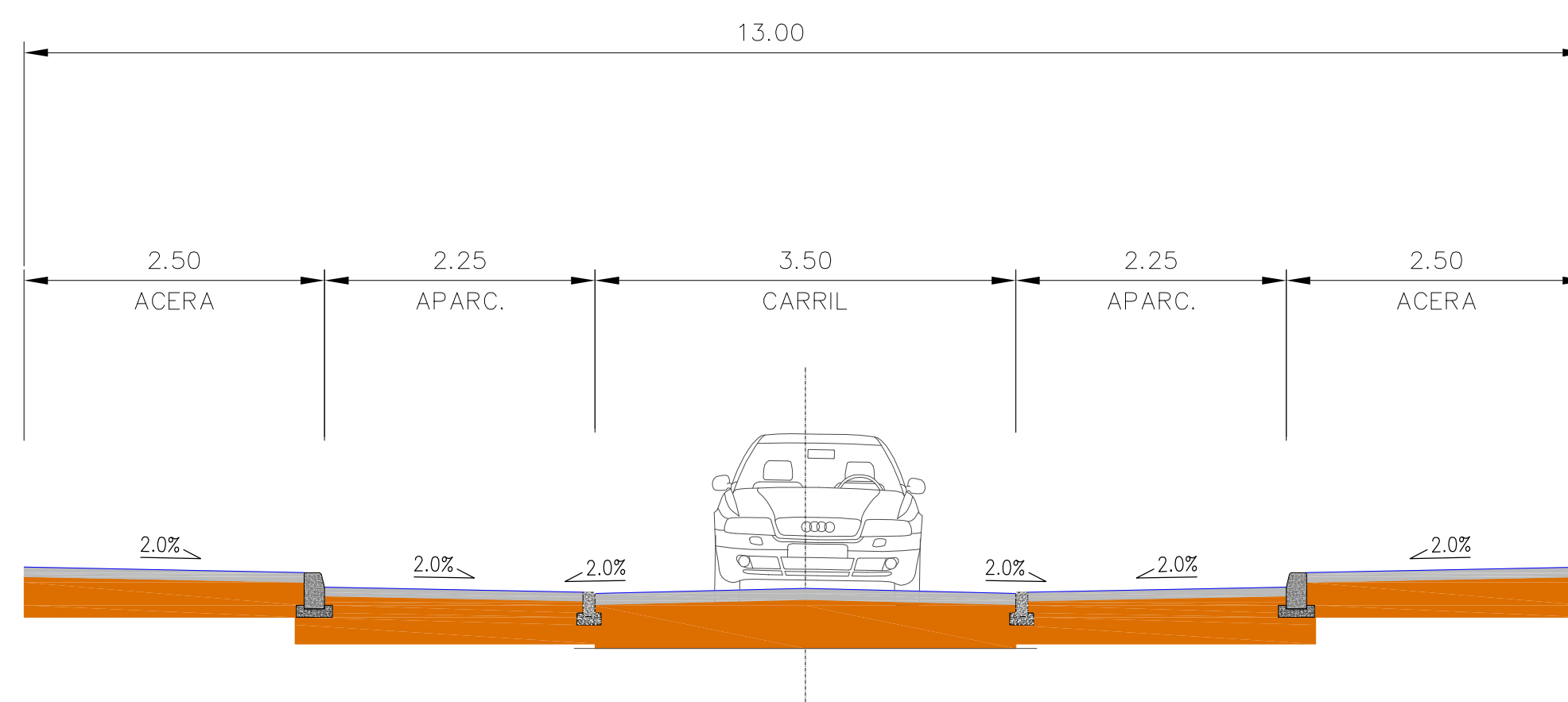
SECCION TIPO VIAL TERCIARIO D
