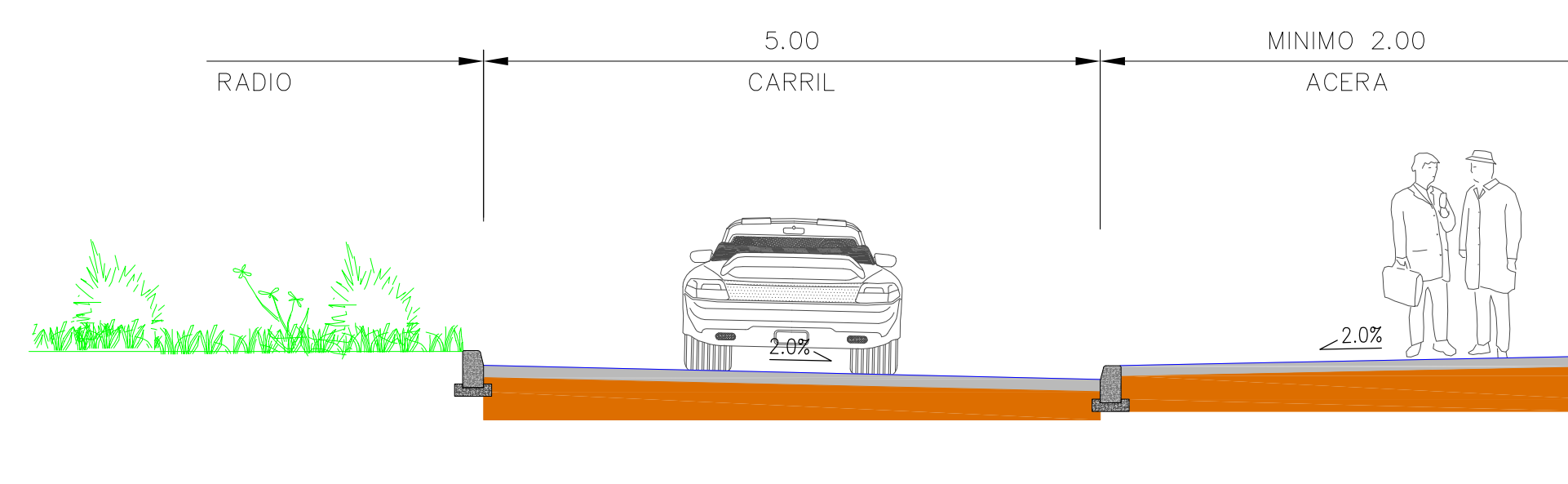
SECCION TIPO EN GLORIETAS CON UN CARRIL
