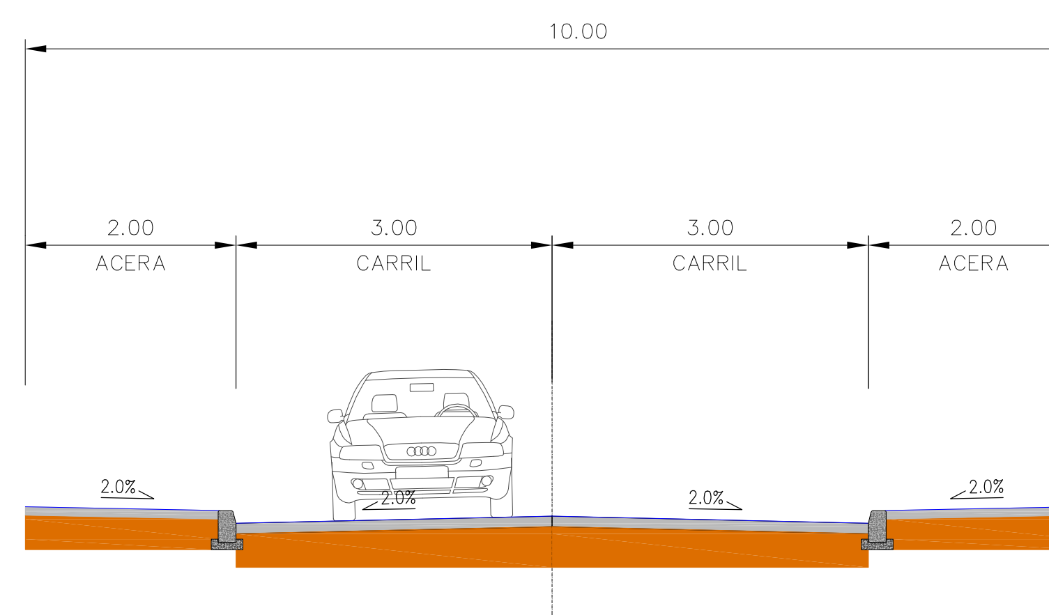
SECCION TIPO VIAL ESPECIAL B
