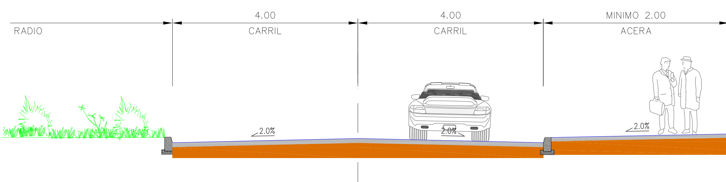
SECCION TIPO EN GLORIETAS DE DOBLE CARRIL
