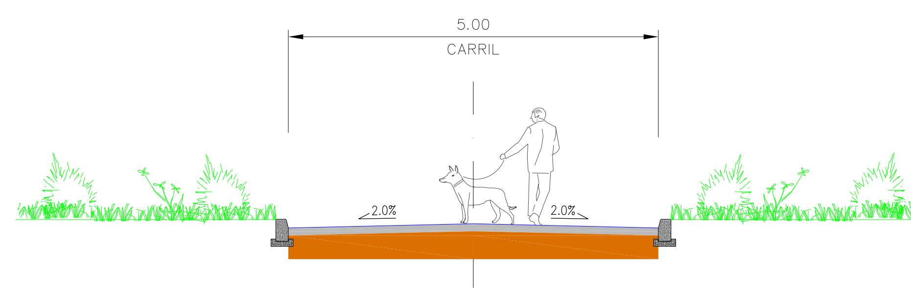
SECCION TIPO VIAL PEATONAL Y VIAL COMPARTIDO B
