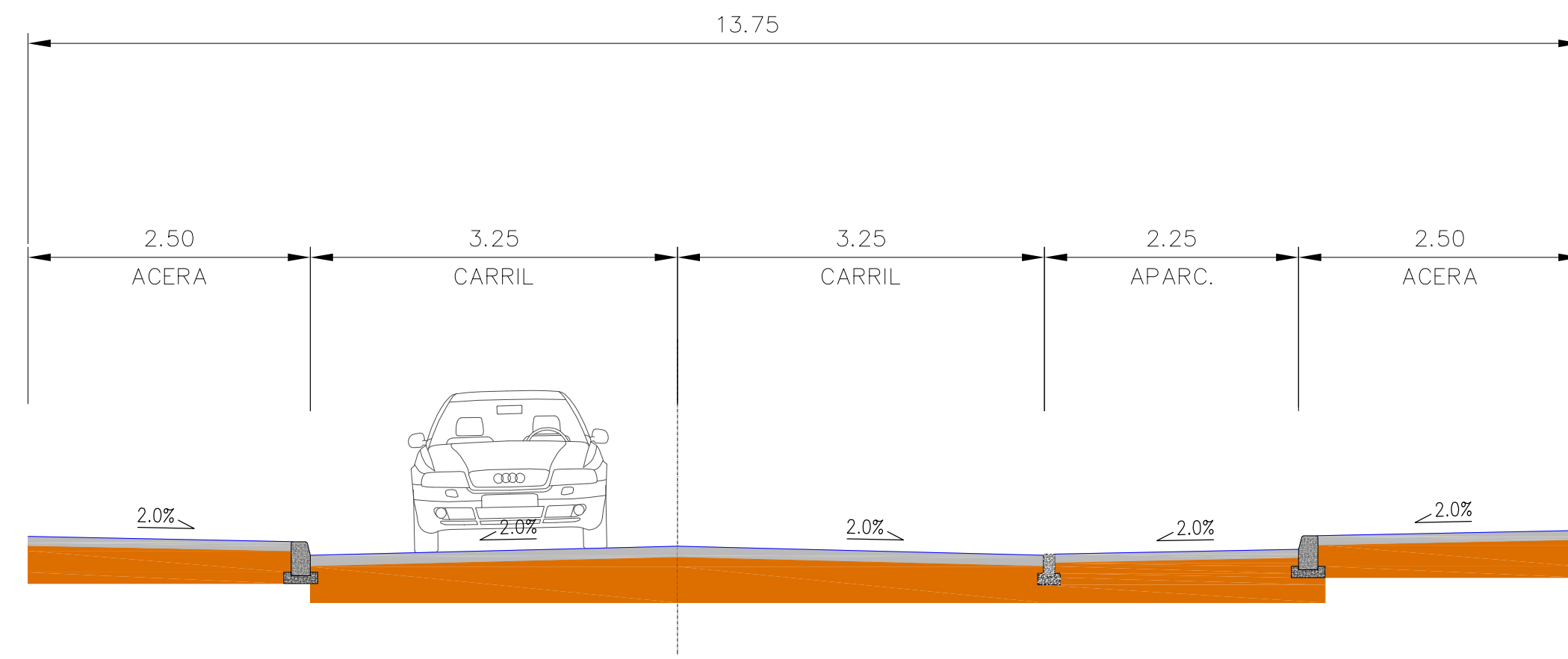
SECCION TIPO VIAL TERCIARIO C
