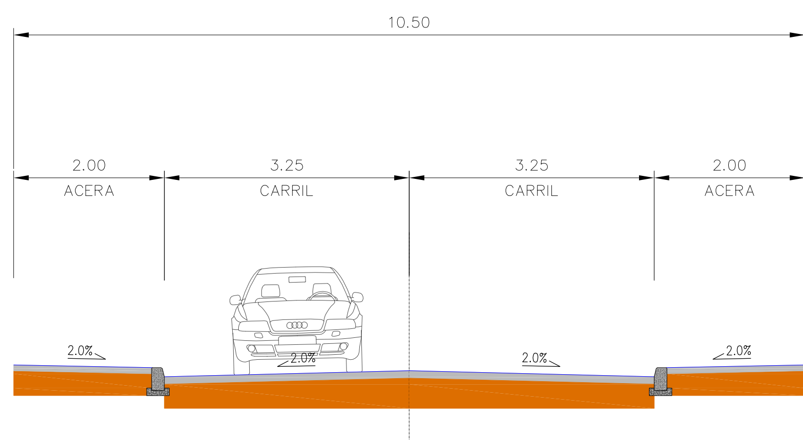
SECCION TIPO VIAL ESPECIAL A
